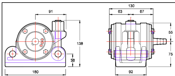
VAQ-75 & 120 mit QR-2 Schnellspannvorrichtung
