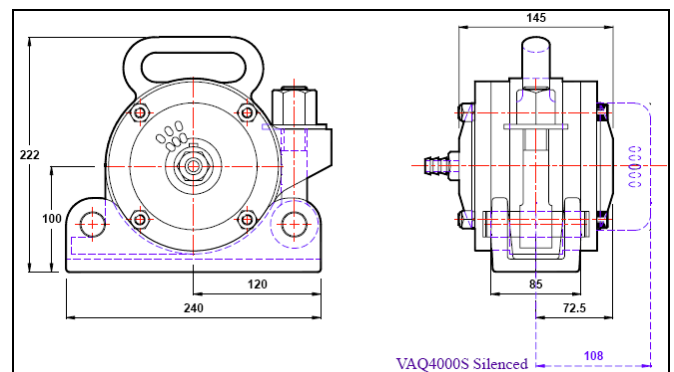
VAQ-2500, 4000, 4500 & 6000 mit QR-4 Schnellspannvorr.
